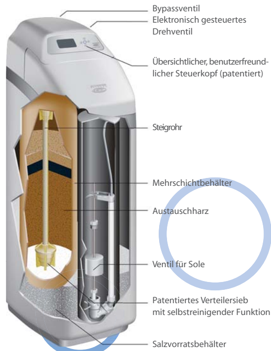
EcoWater Systems Enthärtungsanlage
